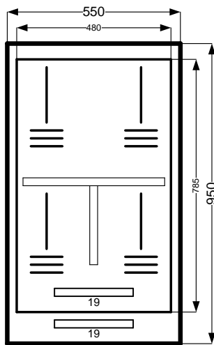
A 2.03 Wechseltafel 785 x 480 mm mit Schrank 950 x 550 x 225 mm
